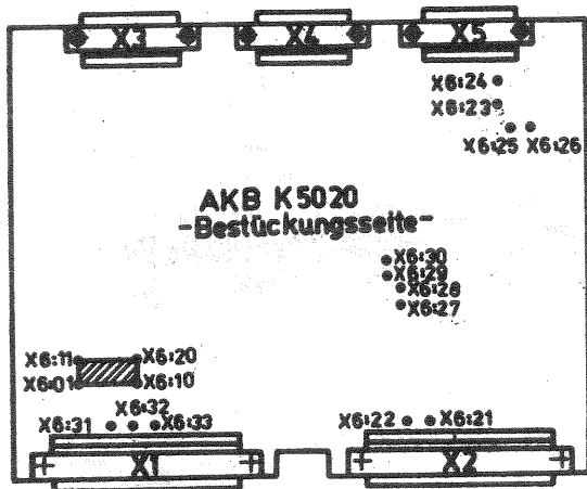
Abb. 1 | Lage der Wickelstifte
