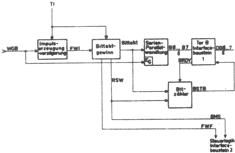
Abb. 3 Eingabesteuerung
